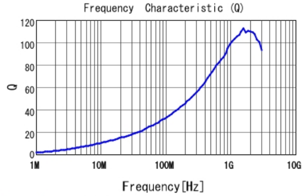
LQW18AN10NJ8Z Q
