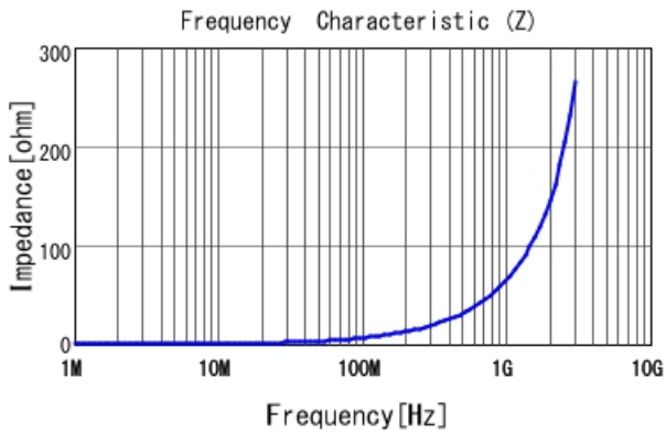
LQW18AN10NJ8Z |Z|
