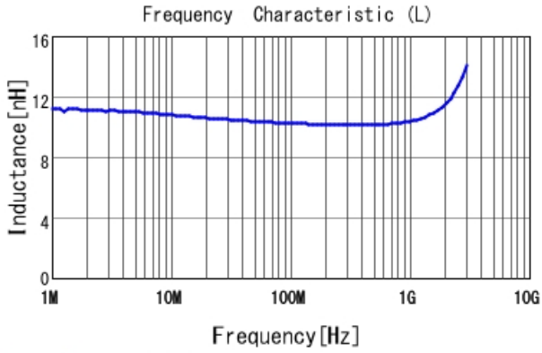
LQW18AN10NJ8Z L
