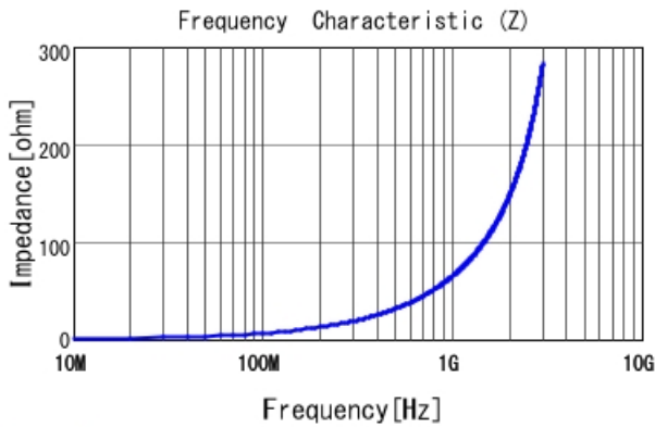
LQW18AS10NG0Z |Z|
