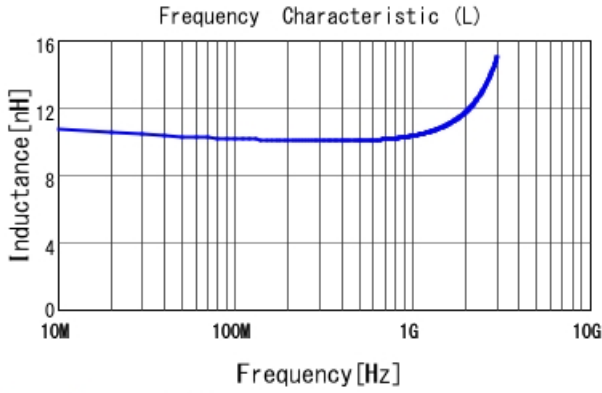
LQW18AS10NG0Z L
