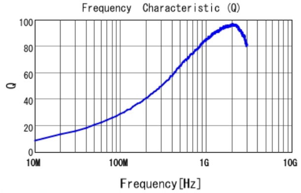
LQW18AS10NG0Z Q
