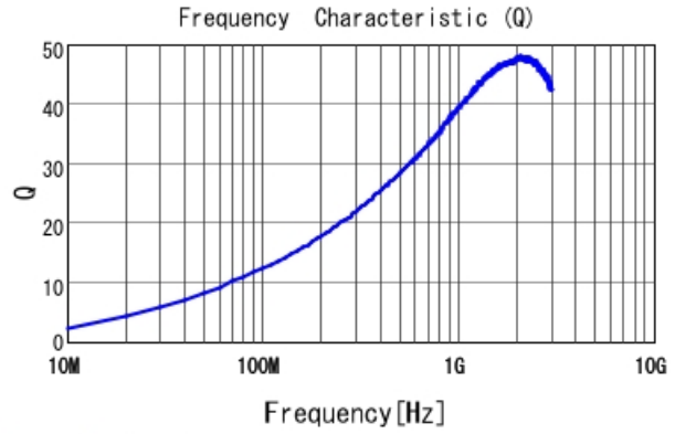
LQP03HQ10NH02 Q
