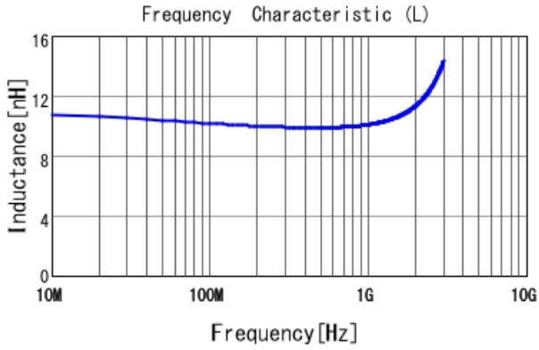
LQP03HQ10NH02 L
