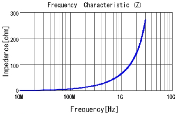
LQP03HQ10NH02 |Z|
