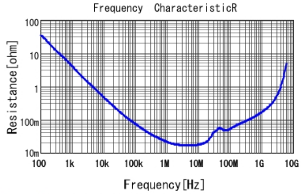
GCJ188R71C224KA01 R DCOV, 25degC
