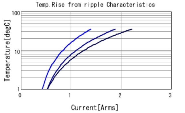
GCJ188R71C224KA01 Temp. rise — 300kHz — 600
