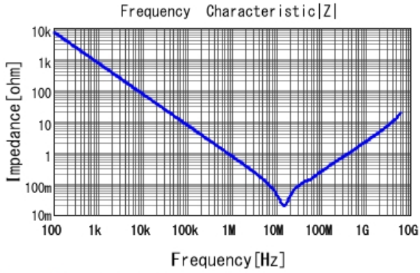
GCJ188R71C224KA01 |Z| DCOV, 25degC
