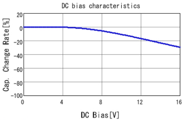
GCJ188R71C224KA01 C-DC bias capchange, 25.0degC, A
