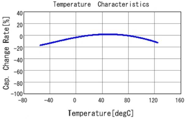
GCM155C71A474KE36 C-Temp. capchange, DCO. 0V, ACO. 2
