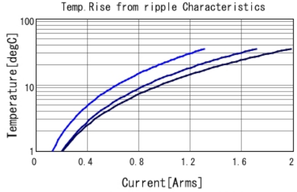
GCM155C71A474KE36 Temp. rise — 200kHz — 500
