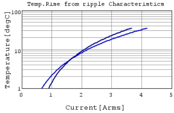
GCM21BR71H105KA03 Temp.rise — 500kHz
