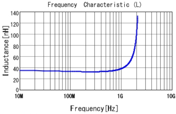
LQG15WZ33NH02 L
