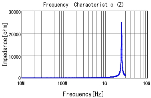
LQG15WZ33NH02 |Z|
