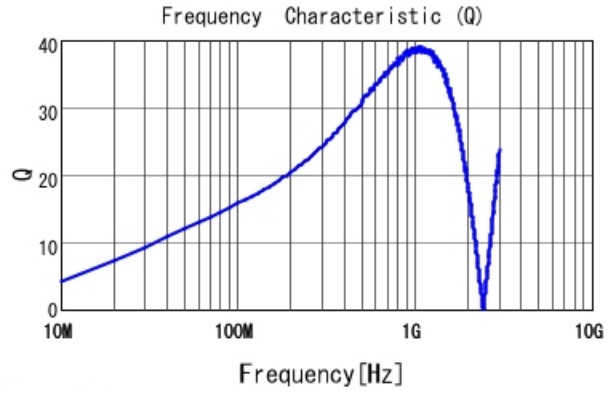
LQG15WZ33NH02 Q
