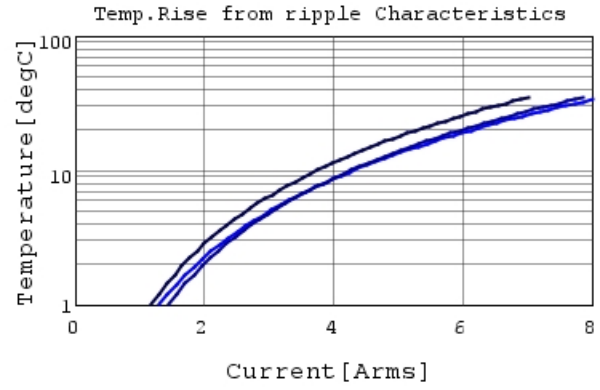
GRM32ER60G337ME05 Temp.rise — 50kHz
