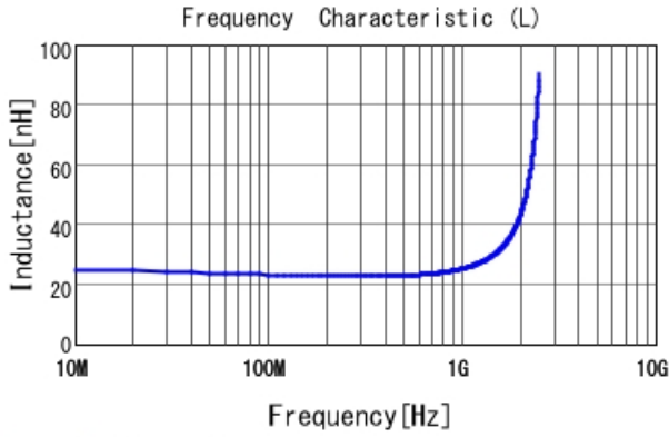
LQG15WH23NG02 L
