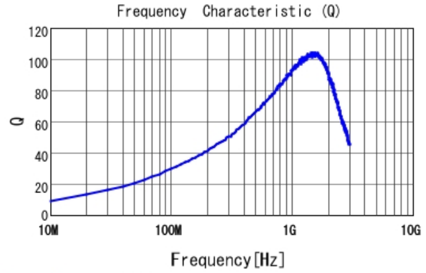
LQW18AN22NJ0Z Q
