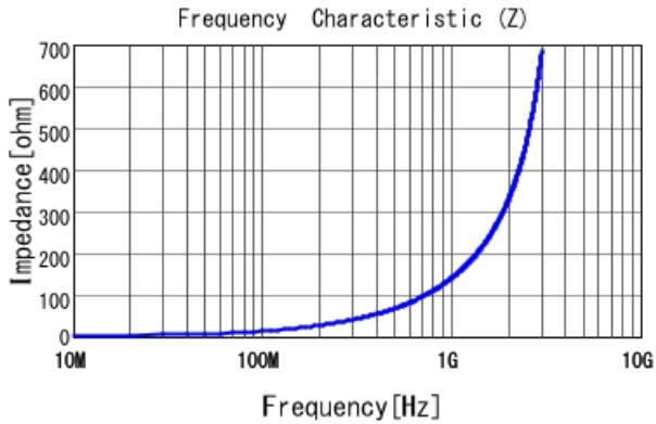
LQW18AN22NJ0Z |Z|
