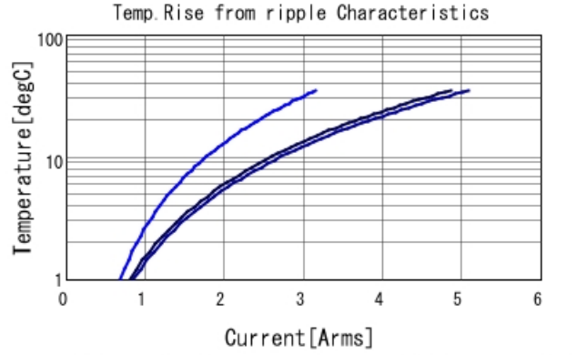
GRM32MB11C225KA01 Temp. rise — 100kHz — 500
