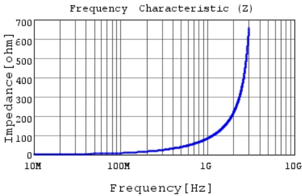
LQG15WZ13NH02 |Z|
