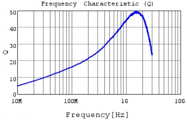
LQG15WZ13NH02 Q
