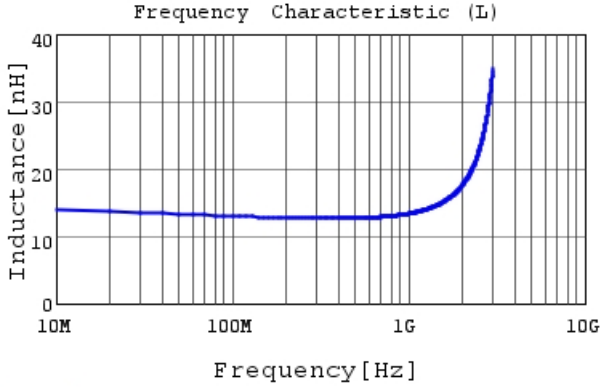
LQG15WZ13NH02 L
