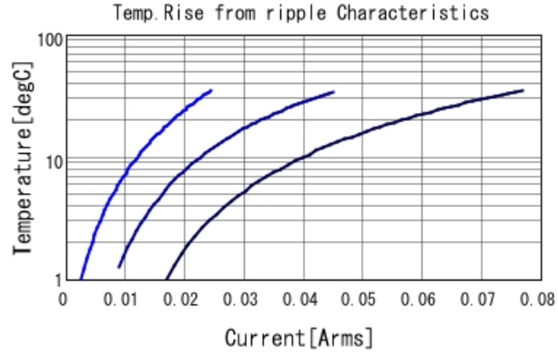
GRM31BR73A471KW01 Temp. rise — 30kHz — 100kl
