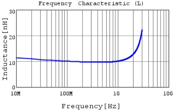
LQG15HZ10NG02 L
