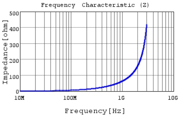
LQG15HZ10NG02 |Z|
