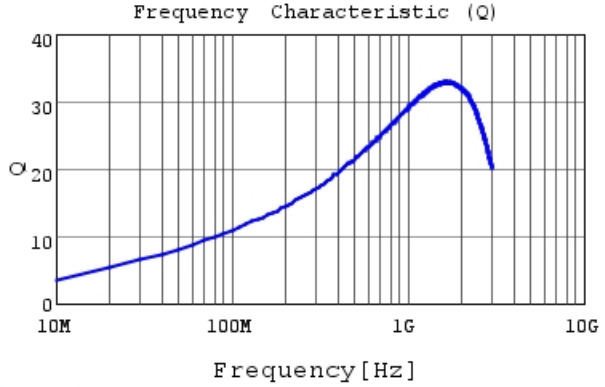
LQG15HZ10NG02 Q
