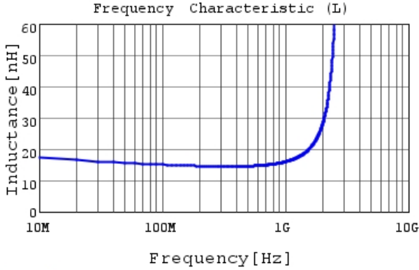
LQG15HZ15NG02 L
