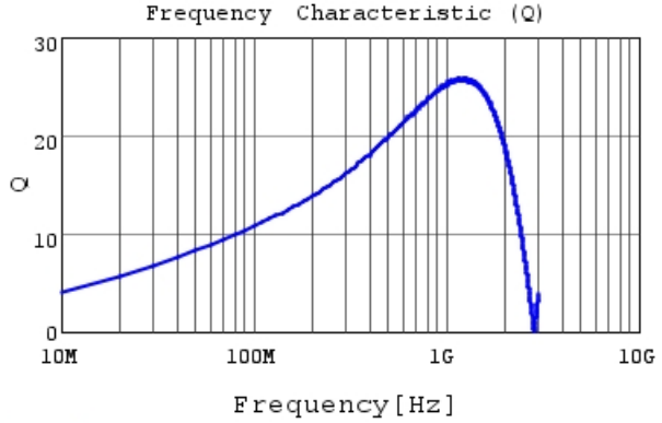
LQG15HZ15NG02 Q
