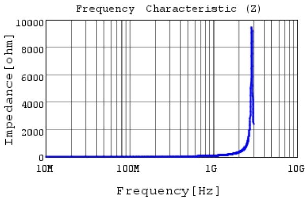
LQG15HZ15NG02 |Z|
