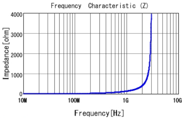
LQG15WH20NH02 |Z|
