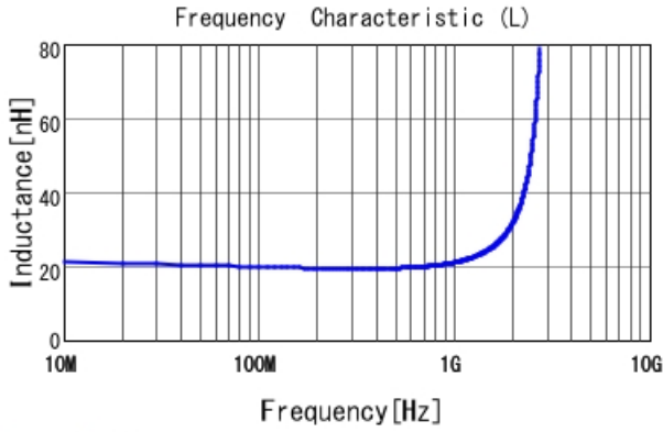
LQG15WH20NH02 L
