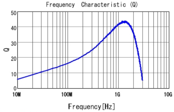
LQG15WH20NH02 Q
