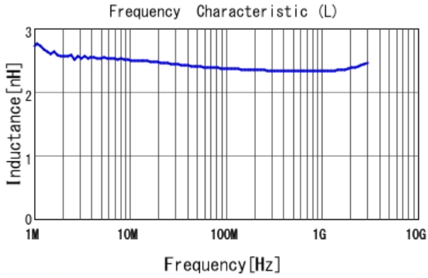
LQW15AN2N4B80 L
