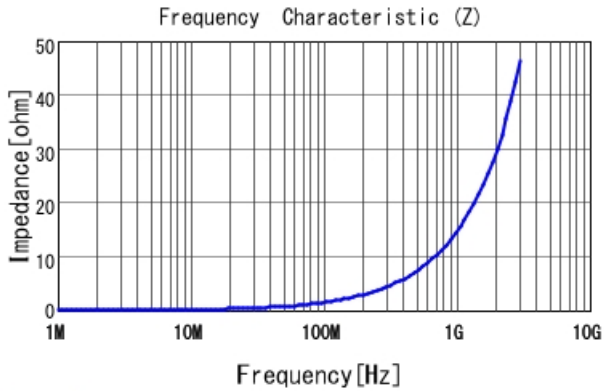
LQW15AN2N4B80 |Z|
