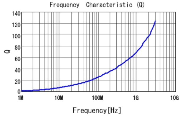
LQW15AN2N4B80 Q
