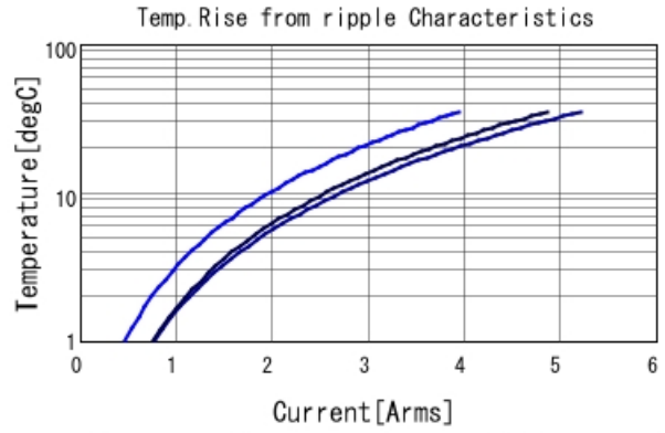
GRM31CC72A475KE11 Temp. rise — 100kHz — 500
