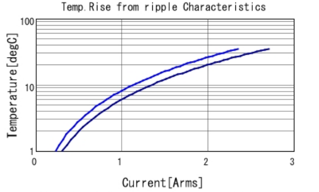
GRM185R61C105KE44 Temp. rise — 500kHz — 1MHz
