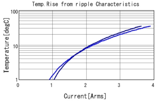
GCJ21BR71H105KA01 Temp. rise — 500kHz — 1MHz
