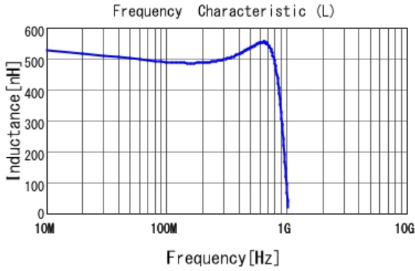
LQW15CAR50K00 L
