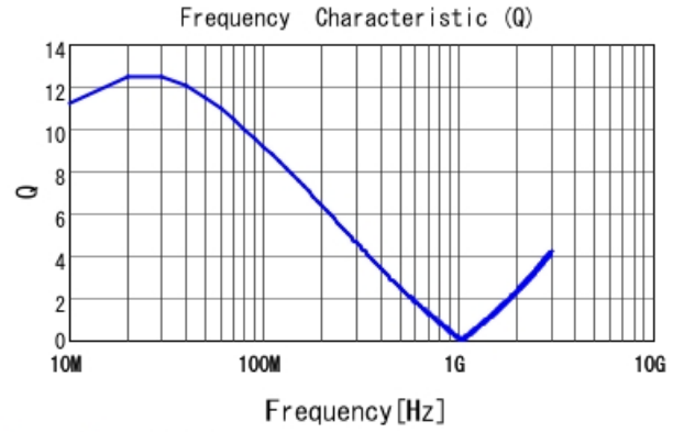
LQW15CAR50K00 Q
