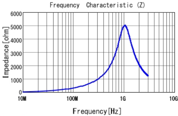
LQW15CAR50K00 |Z|
