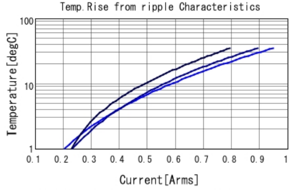
GRM1555C1H100JA01 Temp. rise — 700MHz — 1GHz
