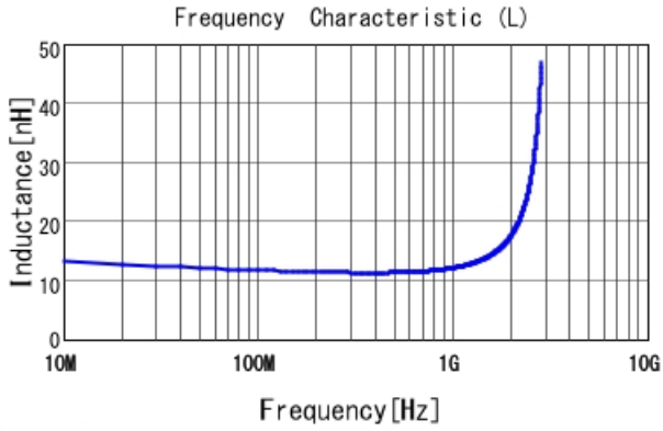
LQG15HH12NH02 L
