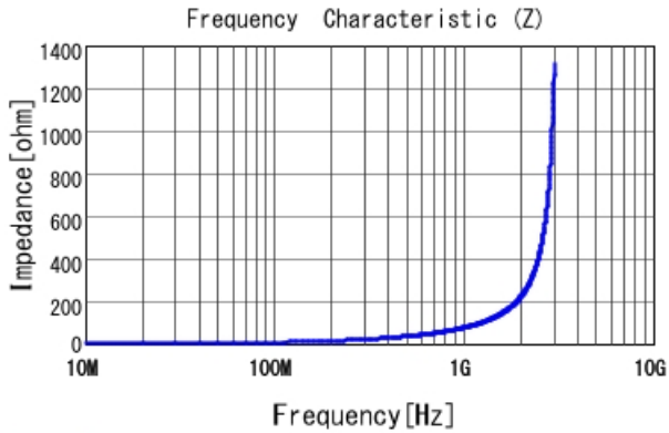
LQG15HH12NH02 |Z|
