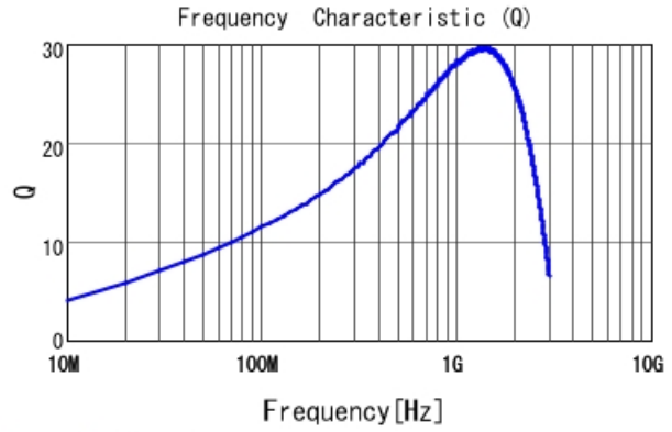
LQG15HH12NH02 Q
