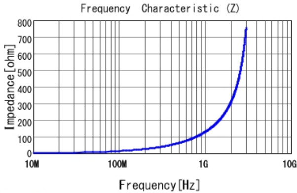
LQP02HQ20NH02 |Z|
