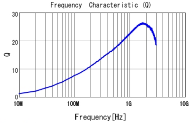
LQP02HQ20NH02 Q
