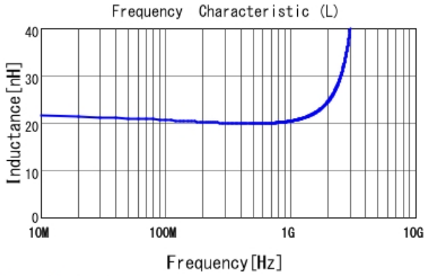
LQP02HQ20NH02 L
