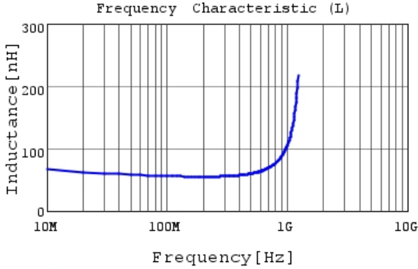
LQG15HN56NH02 L
