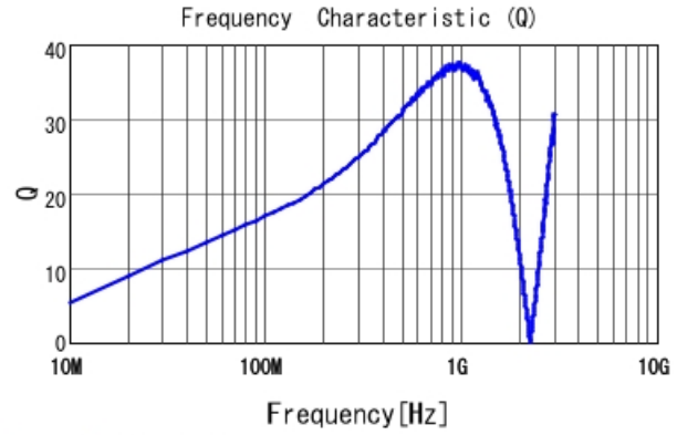
LQG15WZ36NJ02 Q
