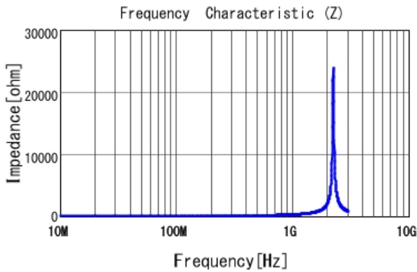
LQG15WZ36NJ02 |Z|
