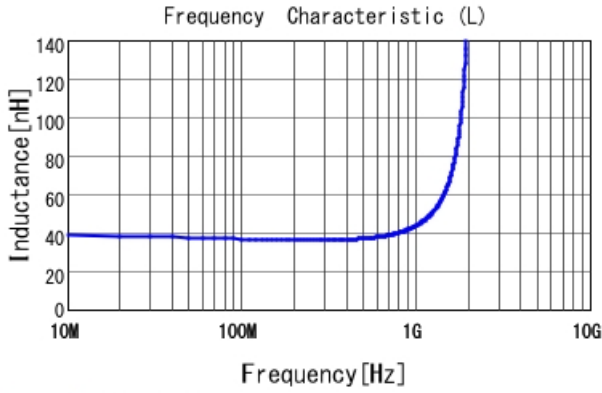
LQG15WZ36NJ02 L
