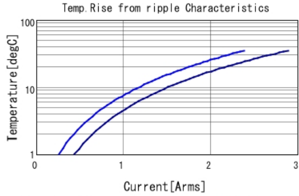
GRM155B31E105KA12 Temp. rise ■ 500kHz ■ 1MHz
