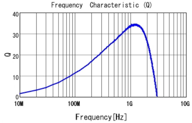
LQP03HQ27NH02 Q
