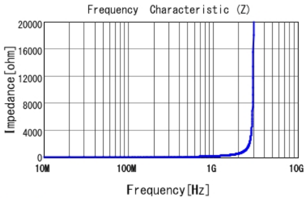
LQP03HQ27NH02 |Z|
