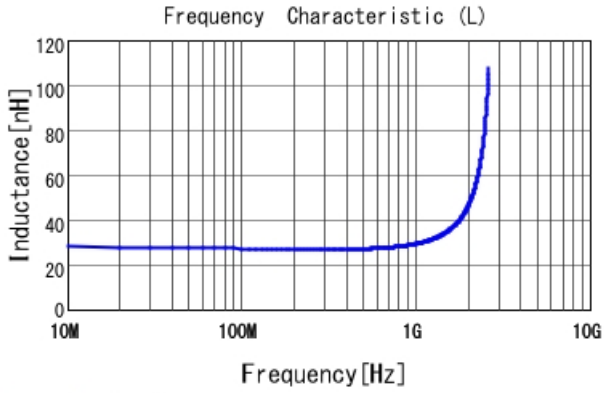
LQP03HQ27NH02 L
