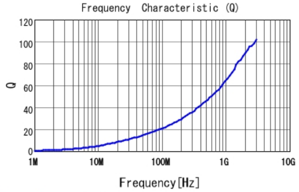
LQW15AN4N7G8Z Q
