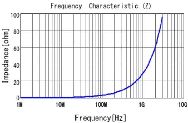
LQW15AN4N7G8Z |Z|
