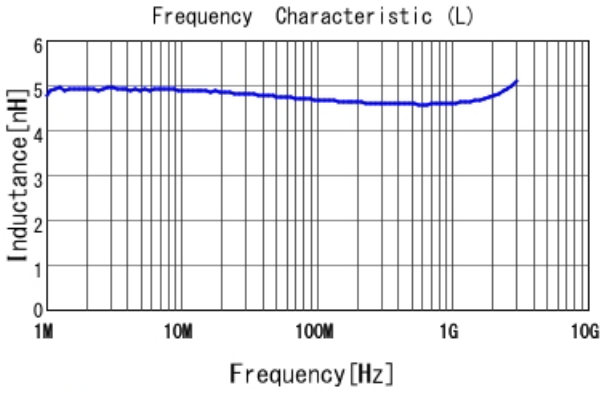
LQW15AN4N7G8Z L
