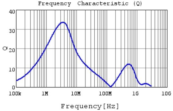
LQH2MPZ2R2MGR Q
