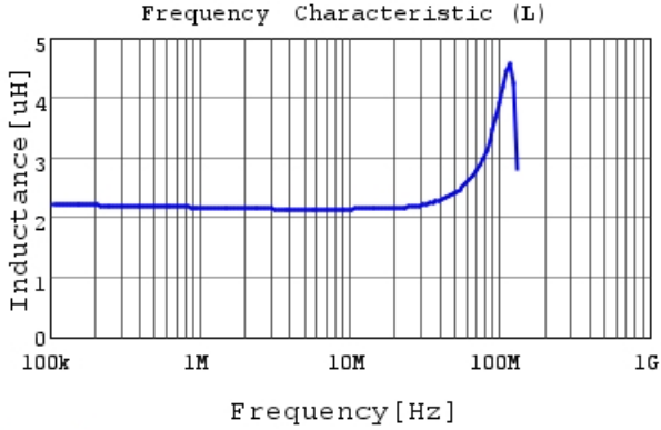
LQH2MPZ2R2MGR L
