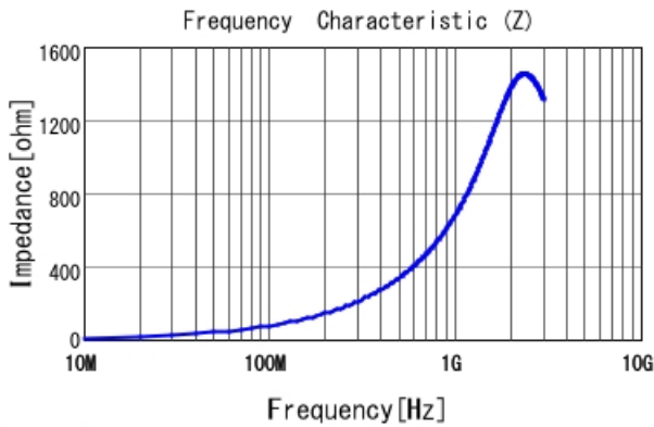
LQW04CAR12K00 |Z|
