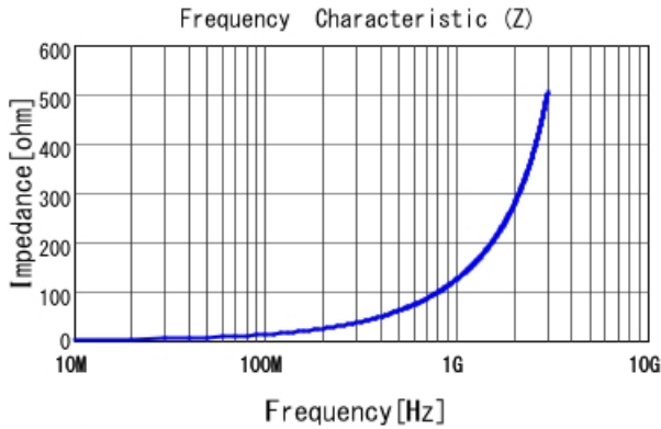
LQW15AN20NG0Z |Z|
