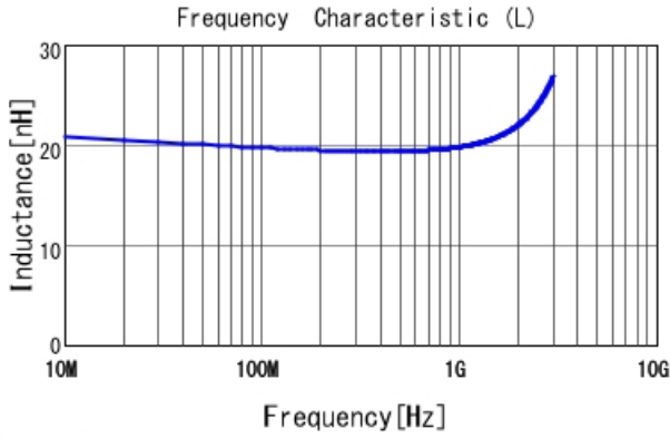
LQW15AN20NG0Z L
