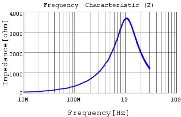
LQW18CNR56J0Z |Z|
