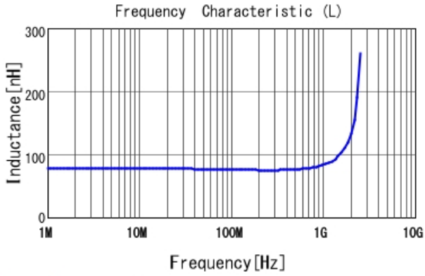
LQW15AN75NG80 L
