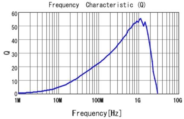
LQW15AN75NG80 Q
