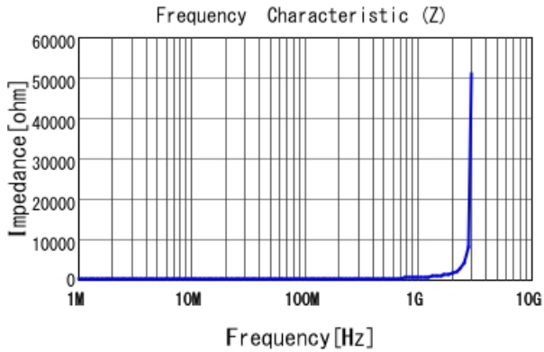
LQW15AN75NG80 |Z|
