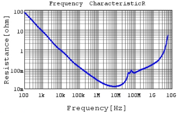
GCM188L81H104KA57 R DCOV, 25degC
