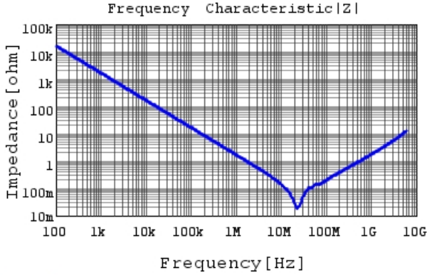
GCM188L81H104KA57 |Z| DCOV, 25degC
