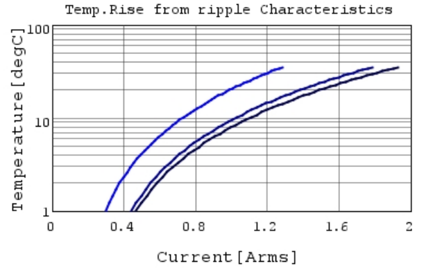
GCM188L81H104KA57 Temp.rise — 400kHz —
