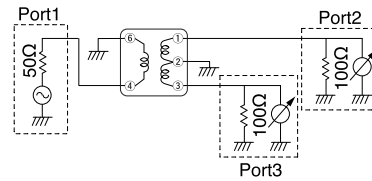
2) #617PT-1664 (Impedance Ratio/阻抗比=50Ω:200Ω)
