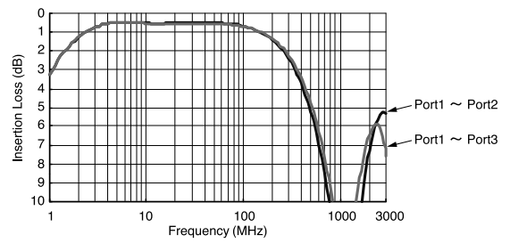
2) #617PT-1664 (Impedance Ratio/阻抗比=50Ω:200Ω)
