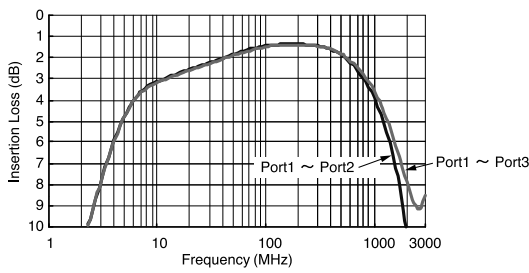
1) #617PT-1667 (Impedance Ratio/阻抗比=50Ω:200Ω)
