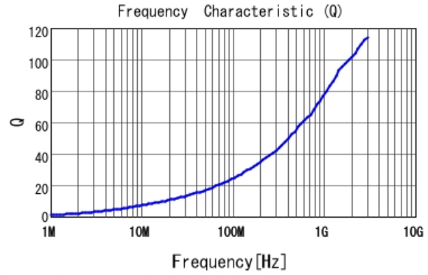
LQW15AN5N5D8Z Q
