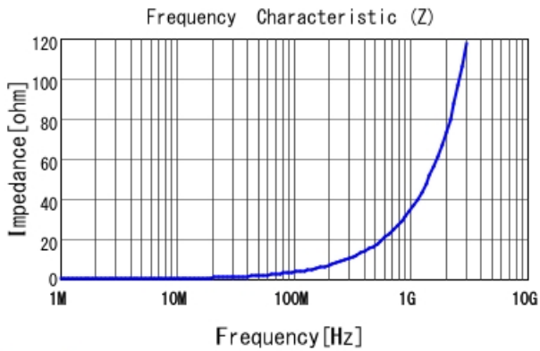
LQW15AN5N5D8Z |Z|
