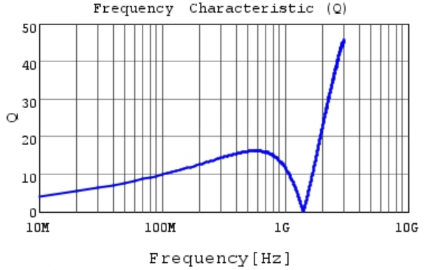
LQG15HN56NJ02 Q
