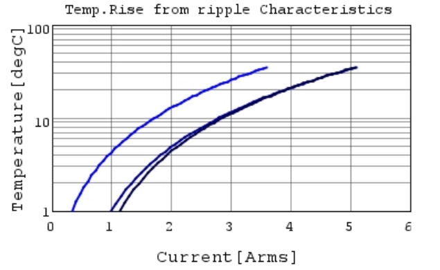
GRM188B30J106ME47 Temp.rise — 80kHz —
