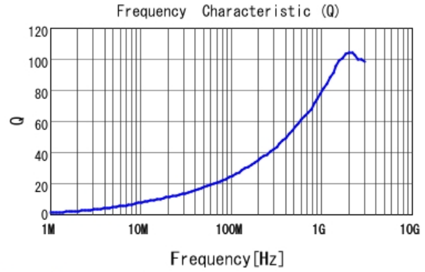
LQW15AN6N2D80 Q
