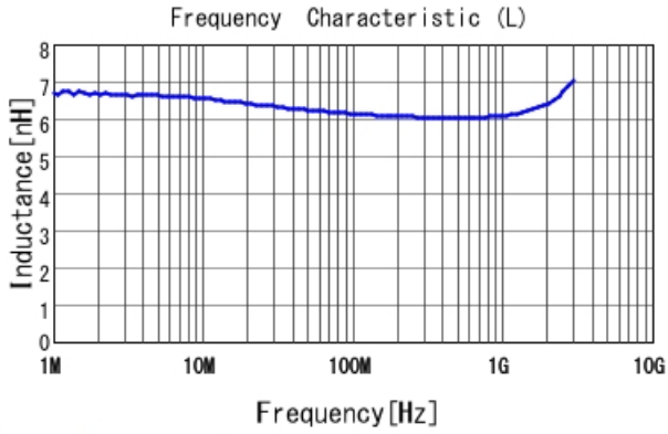
LQW15AN6N2D80 L
