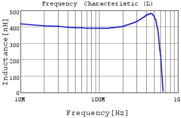
LQW15CNR39K1Z L
