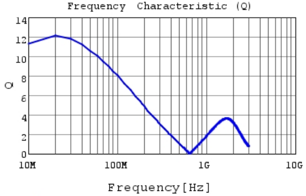
LQW15CNR39K1Z Q
