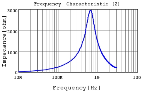
LQW15CNR39K1Z |Z|
