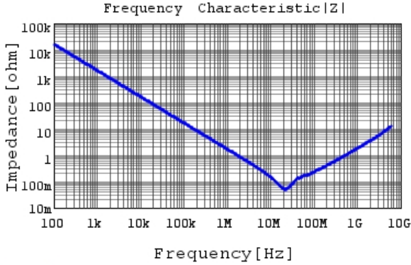
GCJ188R71H104KA12 |Z| DCOV,25degC
