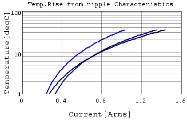
GCJ188R71H104KA12 Temp.rise — 400kHz —
