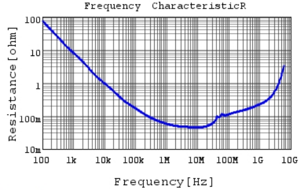
GCJ188R71H104KA12 R DCOV,25degC
