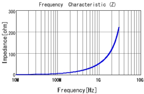
LQP03TG8N2H02 |Z|
