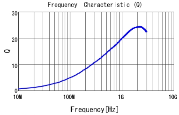
LQP03TG8N2H02 Q
