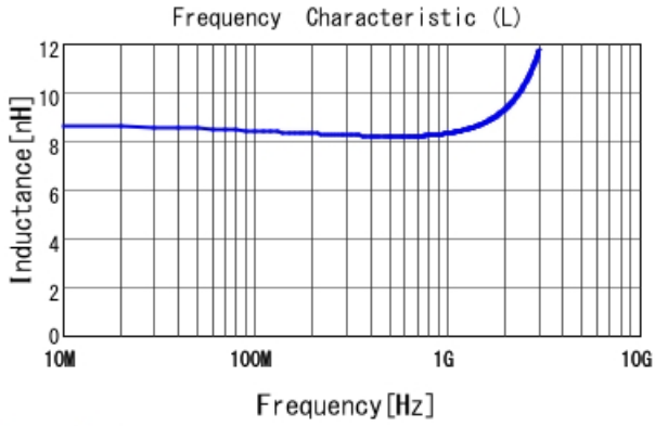
LQP03TG8N2H02 L
