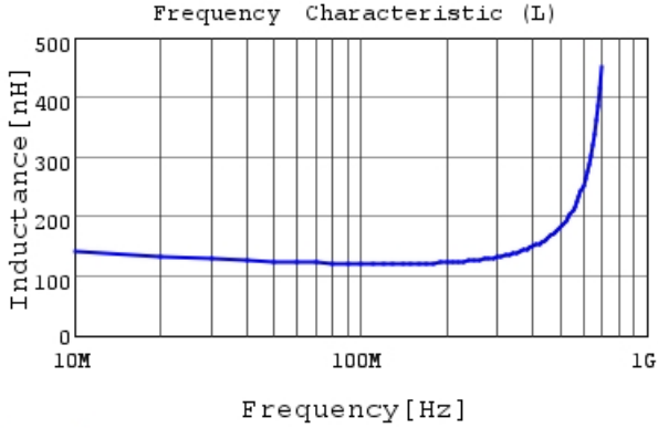
LQG15HNR12J02 L
