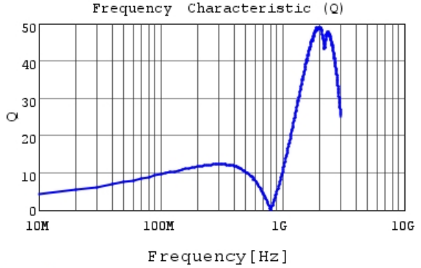
LQG15HNR12J02 Q
