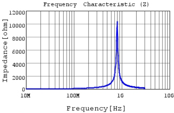
LQG15HNR12J02 |Z|
