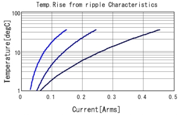
GRM31CR72J153KW03 Temp. rise — 30kHz — 100kHz
