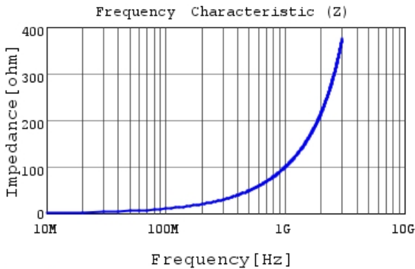
LQW15AN16NG0Z |Z|
