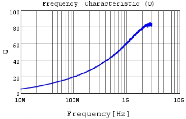
LQW15AN16NG0Z Q
