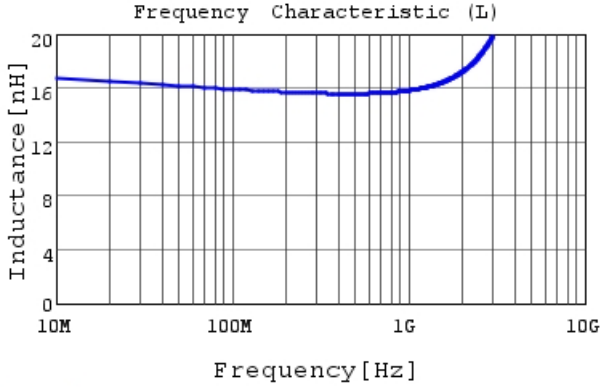
LQW15AN16NG0Z L
