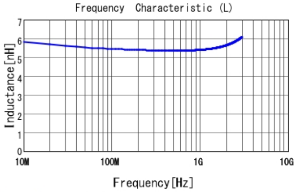
LQW15AN5N4C1Z L
