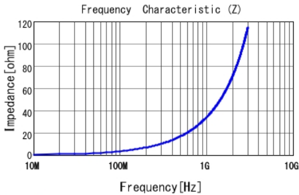
LQW15AN5N4C1Z |Z|
