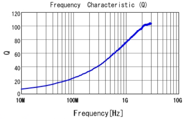
LQW15AN5N4C1Z Q
