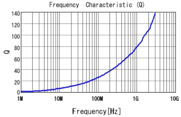
LQW15AN2N3B80 Q
