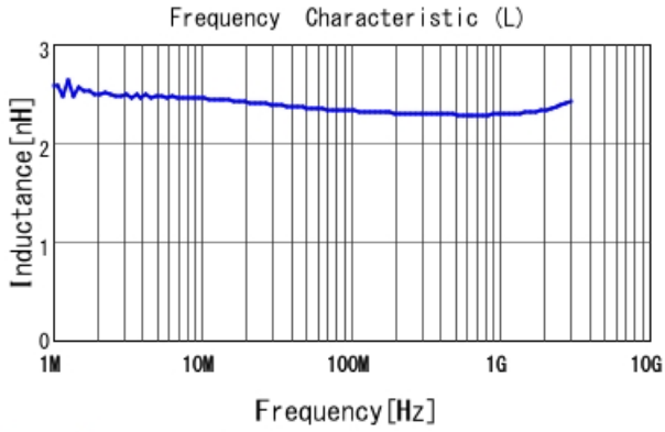
LQW15AN2N3B80 L
