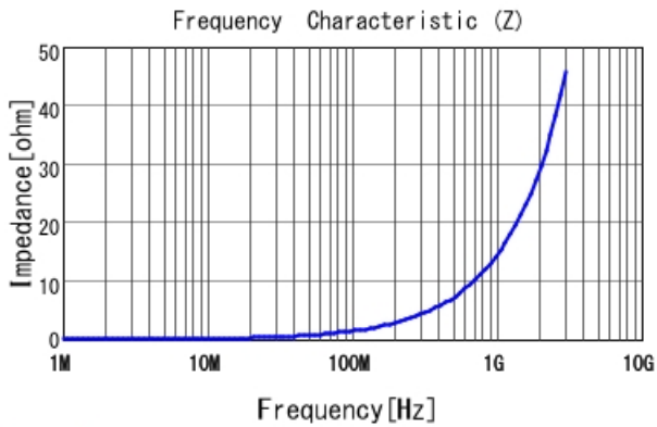
LQW15AN2N3B80 |Z|
