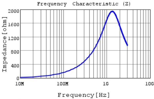
LQW18CNR27J00 |Z|
