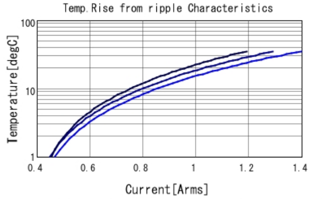
GJM1555C1H270FB01 Temp. rise — 500MHz — 700I
